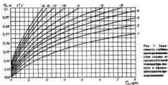
"Рис. 7. Зависимость глубины промораживания слоя осадка от среднесуточной температуры воздуха и продолжительности промораживания"
