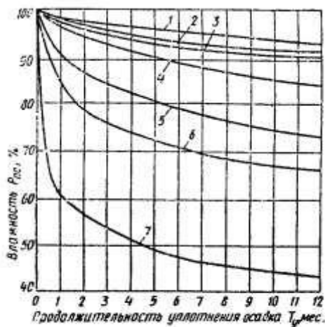
Рис. 3. Средние значения влажности осадка станций осветления и обезвреживания воды при уплотнении до одного года
